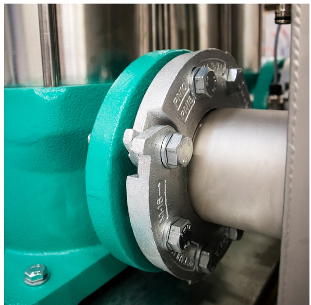
Flanschanschluss montiert.
