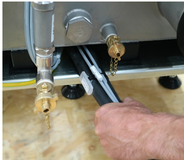
Kabelstrang mittig unter Behälter führen.
