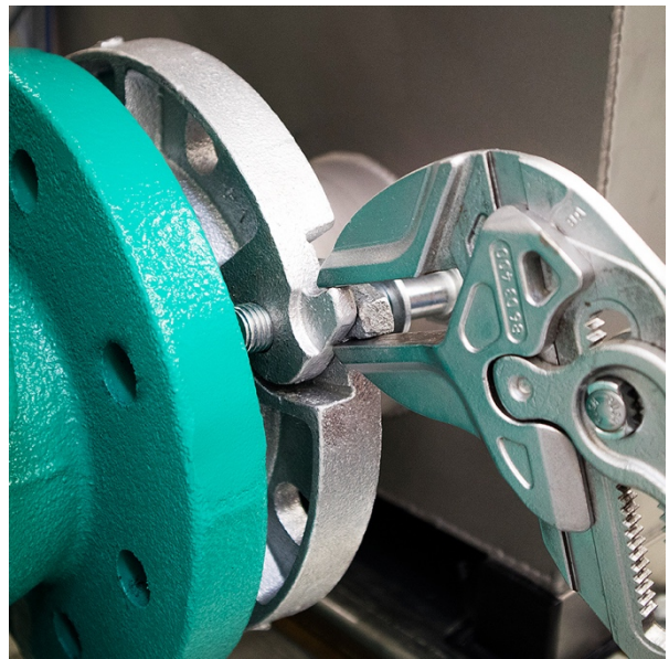
Klappflanschöffnung zum Fixieren drehen.
