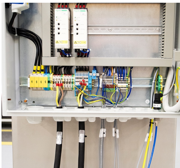
Eingeführte Kabel mit Beschriftung vorn.
