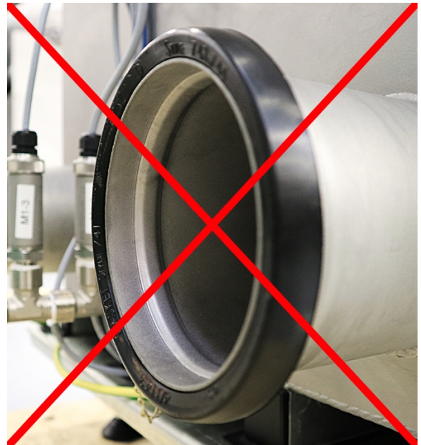
ACHTUNG! Falsch montierte Dichtung.
