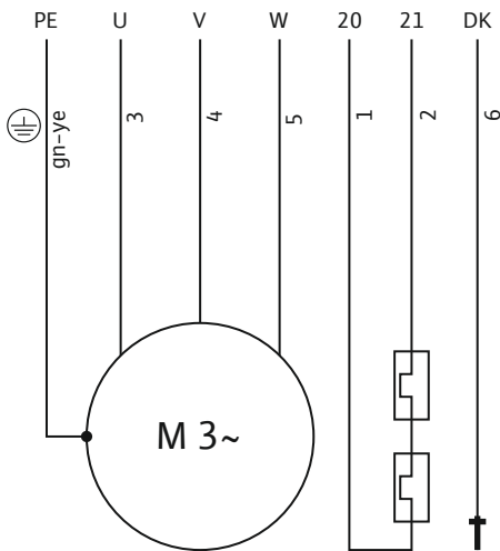
Fig. 8: Комутаційна схема Прямий пуск, біметалевий давач
