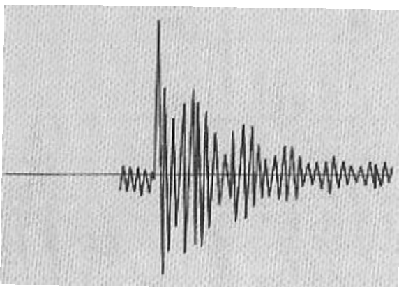
Осциллограмма гидроудара
