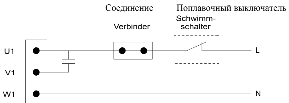
Рисунок 3. Подходит для исполнения EM Подключение поплавочного выключателя (заказывается отдельно) в распределительной коробке электродвигателя
