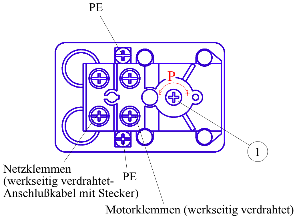
Bild 2 Druckschalter mit fester Differenzdruckeinstellung Ausf \ddot{u} hrung EM
