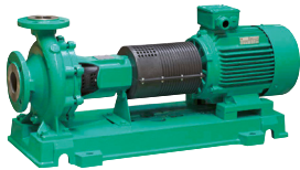
Wilo-CronoNorm-NL Q max. 650 m³/h H max. 150 m
