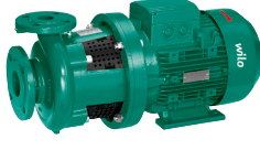
Wilo-CronoBloc-BL Q max. 710 m³/h H max. 104 m
