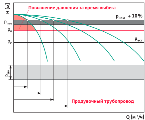
Диаграмма SV
