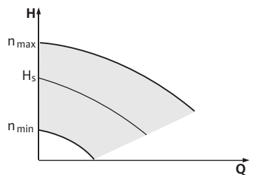
Rys. 41: Tryb sterowania
