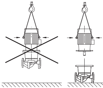
Rys. 8: Transport silnika
