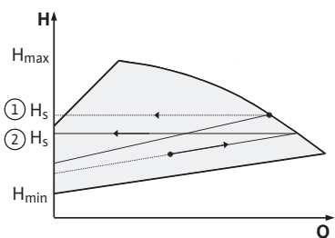
Rys. 40: Regulacja \Delta p-c/\Delta p-v
