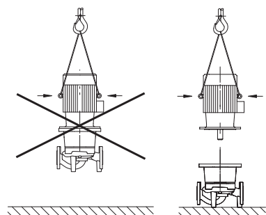
Rys. 20: Transport silnika
