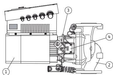
Fig.10: Pompa z pełnym wyposażeniem
