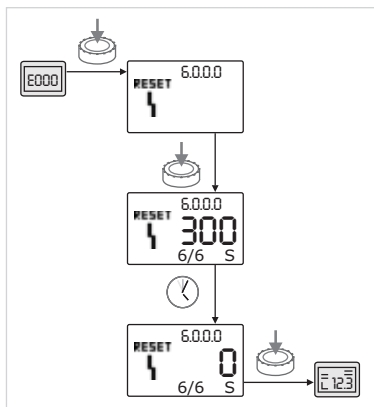
Fig.60: Potwierdzanie błędu typu B (X = Y)
