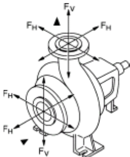
Fig.27: Siły oddziałujące na króćciec
