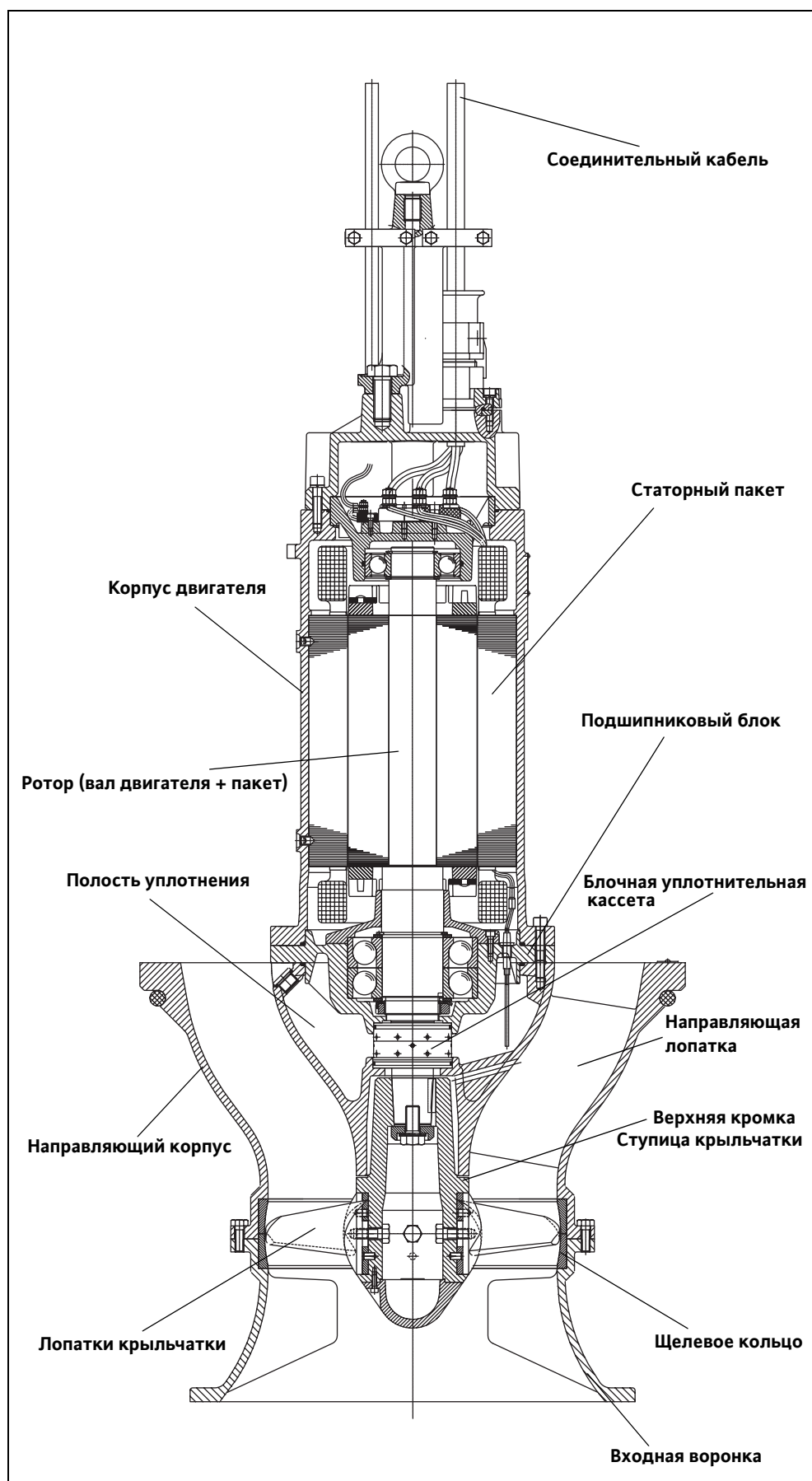
Рис. 3-2: Конструкция оборудования
