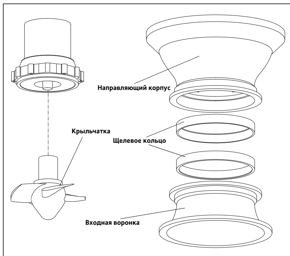
Рис. 3-1: Крыльчатка
