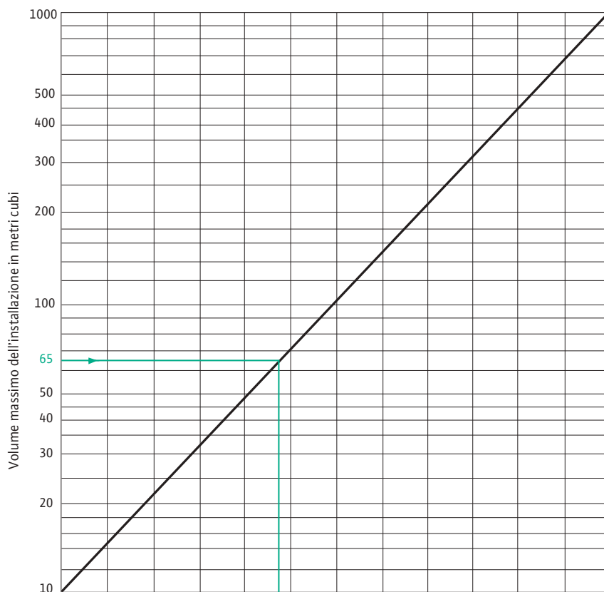
Modello Wilo-SiClean
